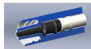
新型ガスケット構造
